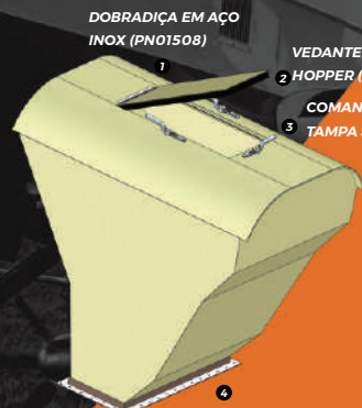
FLANGE DO HOPPER (PN01755) - SEM PORCA FLUTUANTE (PN01756) - COM PORCA FLUTUANTE
