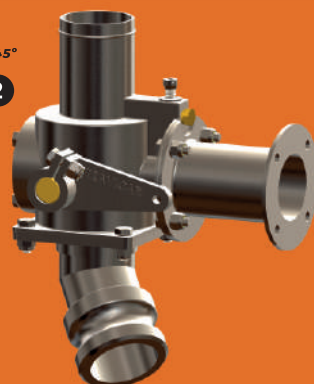
VALVULA CORTE 2" (PN01734)
