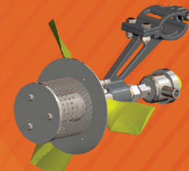
ATOMIZADOR ROTATIVO TELA 75 D125 (PN07165NX)
