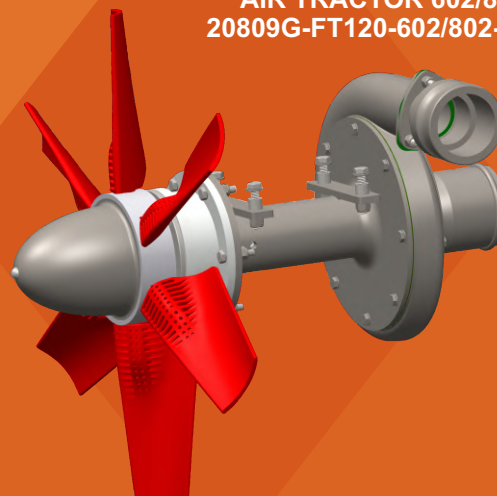
CUBO DE HÉLICE COM 3 POSIÇÕES (PITCH)
