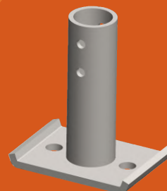
SUPOORTE FIXAÇÃO IPANEMA 203
