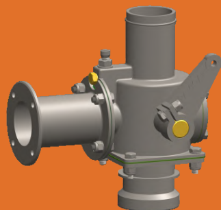
VÁLVULA BY PASS 2" CESSNA (PADRÃO) 01772H7
