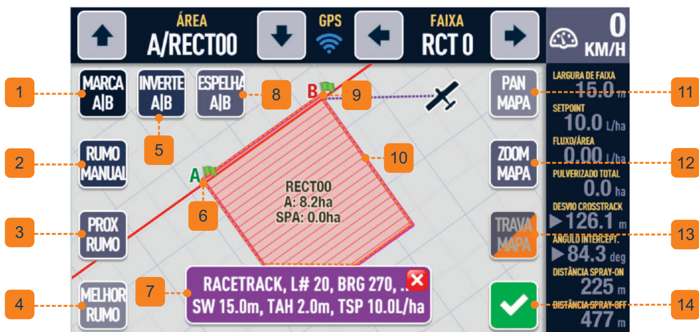
Imagem 40: Tela de Rumo da Área
