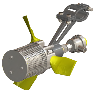
ATOMIZADOR 81mm
