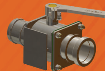
VÁLVULA DE ABASTECIMENTO 2" E (PN01770H7)
