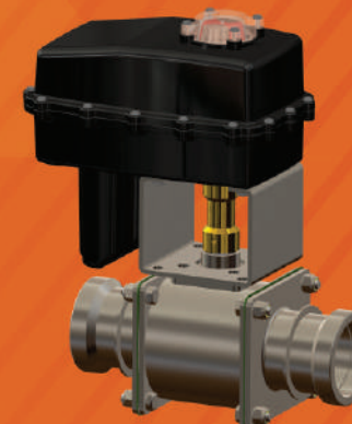
VÁLVULA FLUXÔMETRO 2" (PN - 90232)
