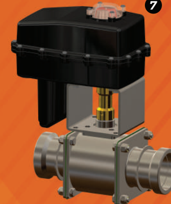
VÁLVULA ON/OFF MANGUEIRA - MANGUEIRA (PN90217/MANGMANG)
