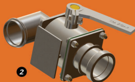
VÁLVULA DE ABASTECIMENTO 2\"/>
