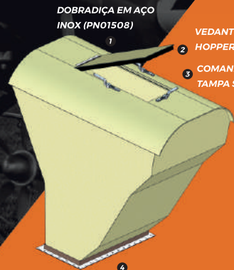
FLANGE DO HOPPER (PN01755) - SEM PORCA FLUTUANTE (PN01756) - COM PORCA FLUTUANTE
